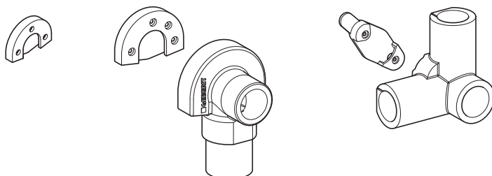
Afbeelding 17: Geberit isolaties voor muurplaten
