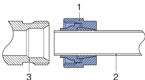
Afbeelding 35: Schroefaansluiting voor Euroconus
