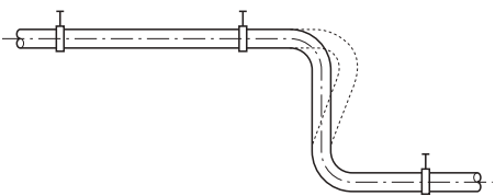
Afbeelding 47: Opname van de lengteverandering \Delta l door de elasticiteit van het leidingsysteem
