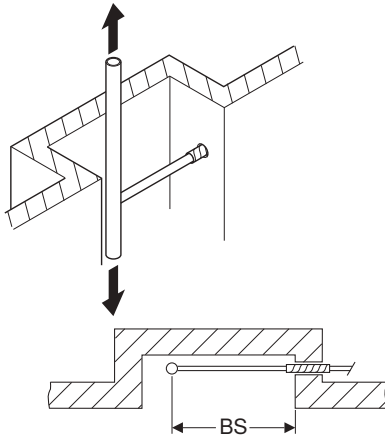
Afbeelding 53: Buigbeen recht, zonder isolatie
