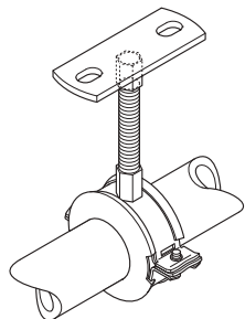
Afbeelding 62: Bevestiging met geïsoleerde beugel
