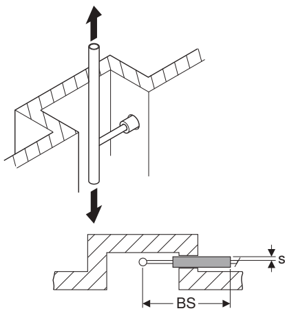
Afbeelding 55: Buigbeen recht, met isolatie
