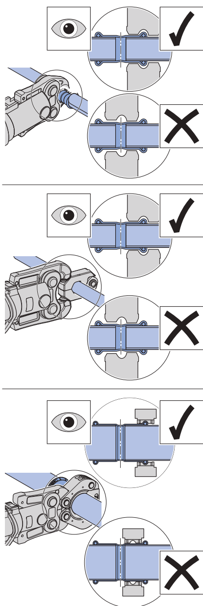
Afbeelding 70: Positionering Geberit Mapress persbek en persketting
