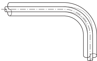
Afbeelding 48: Opname van de lengteverandering \Delta l door comprimeerbare isolatie
