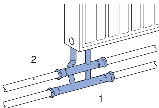
Afbeelding 32: Aansluiting bij opbouwleiding (plint), met aansluiting 4 cm
