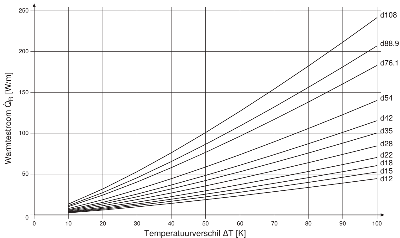
Afbeelding 45: Warmteafgifte voor koperen buizen
