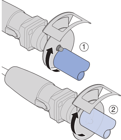
Afbeelding 65: Ontbramen met handontbramer of met elektro-buisontbramer
