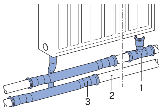
Afbeelding 31: Aansluiting bij opbouwleiding (plint), met afstand tussen aanvoer- en retourleiding
