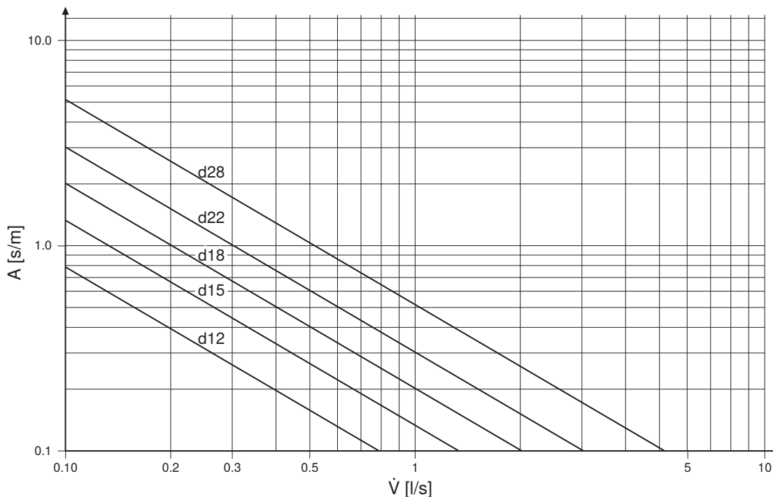
Afbeelding 46: Uitloopfactor A voor Geberit Mapress aanvoerleidingen
