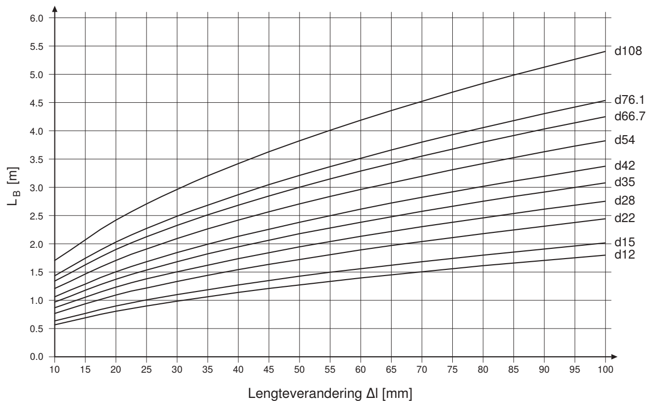
Afbeelding 58: Buigbeenlengte L_B , koperen buizen conform NEN-EN 1057
