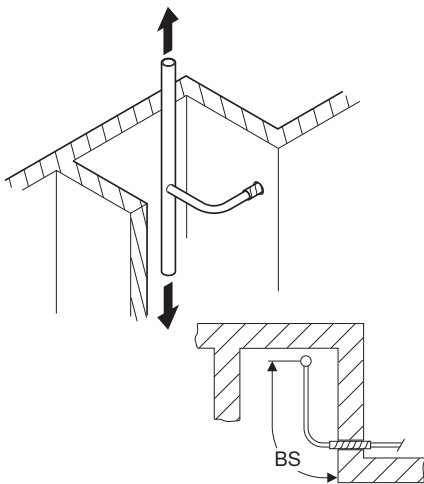
Afbeelding 54: Buigbeen gebogen, zonder isolatie
