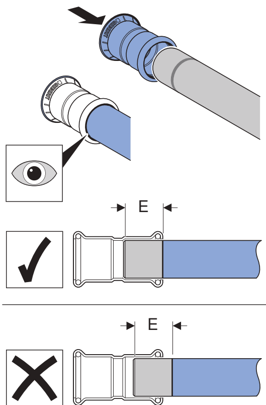
Afbeelding 68: Markering op de buis ter controle van de correcte insteekdiepte
