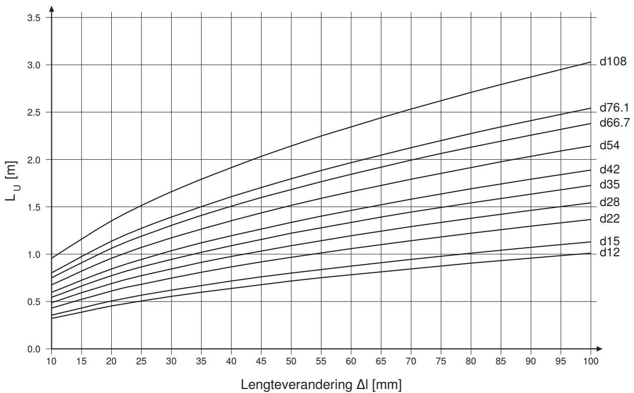
Afbeelding 61: Buigbeenlengte L_U , koperen buizen conform NEN-EN 1057
