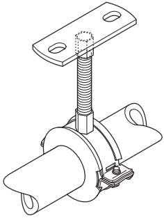
Afbeelding 43: Bevestiging met geïsoleerde beugel
