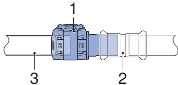
Afbeelding 26: Overgang naar Geberit FlowFit
