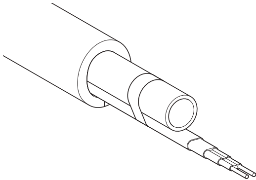
Afbeelding 44: Principe van een warmwaterleiding met warmtelint
