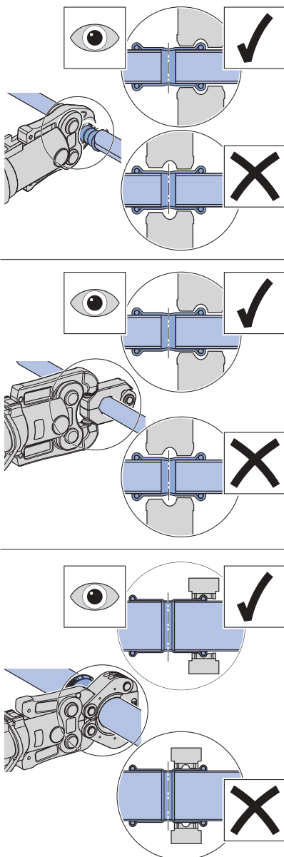
Afbeelding 59: Positionering Geberit Mapress persbek en persketting
