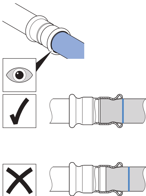
Afbeelding 61: Correcte verpersing
