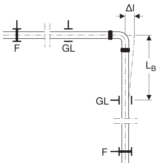
Afbeelding 43: Compensatie van de uitzetting bij richtingsverandering
