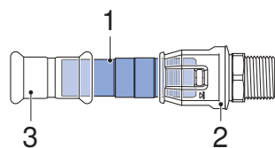
Afbeelding 23: Overgang naar Geberit PushFit
