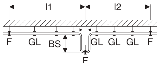
Afbeelding 37: Compensatie van de uitzetting met U-bocht
