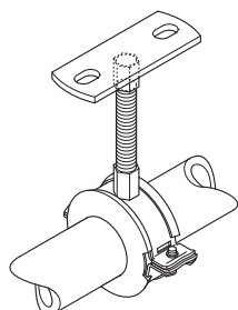
Afbeelding 51: Bevestiging met geïsoleerde beugel
