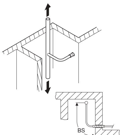
Afbeelding 41: Buigbeen gebogen, zonder isolatie
