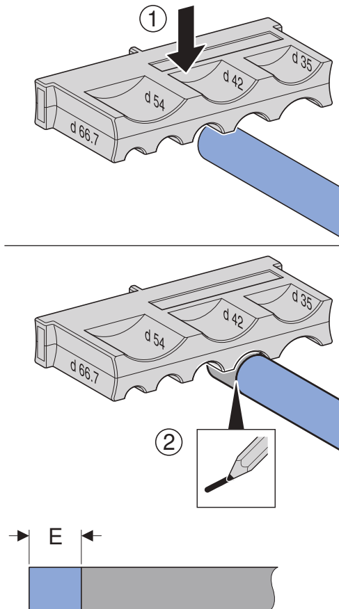
Afbeelding 55: Markering van de insteekdiepte
