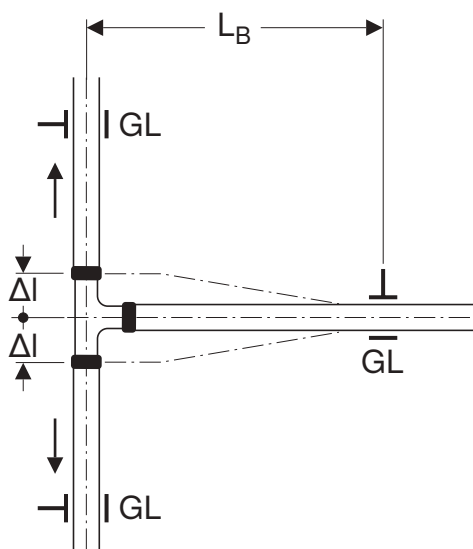
Afbeelding 44: Compensatie van de uitzetting bij aftakking
