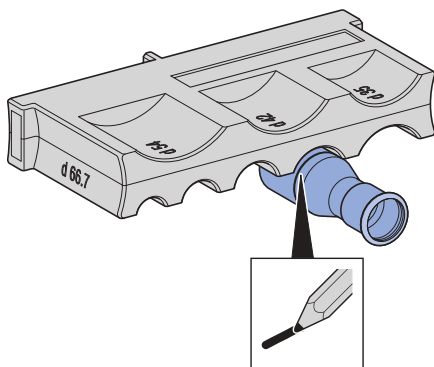
Afbeelding 56: Markering van de insteekdiepte bij fittingen met insteekeinde
