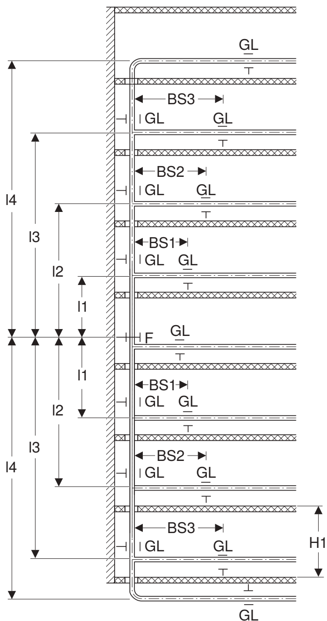
Afbeelding 38: Stijgleiding met fixpunt in het midden: geleiding van de uitzetting naar boven en onderen halveert de buigbeenlengte
