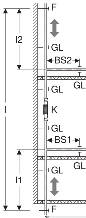
Afbeelding 50: Compensatie van de uitzetting door axiale compensatoren met fixpunt in de onderste etage en in een tussenetage
