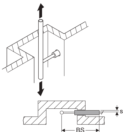
Afbeelding 42: Buigbeen recht, met isolatie
