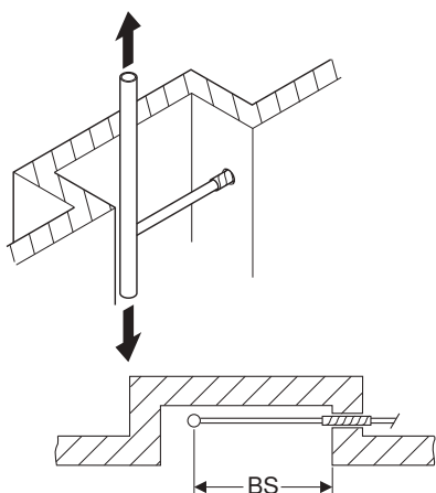
Afbeelding 40: Buigbeen recht, zonder isolatie
