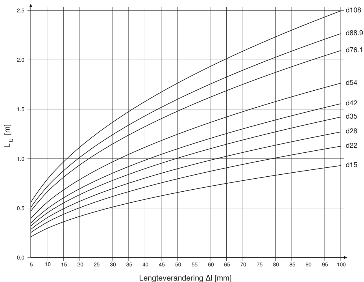
Afbeelding 48: Buigbeenlengte L_U voor Geberit Mapress Therm
