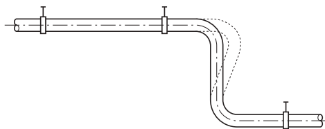
Afbeelding 34: Opname van de lengteverandering \Delta l door de elasticiteit van het leidingsysteem
