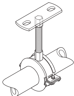
Afbeelding 32: Bevestiging met geïsoleerde beugel
