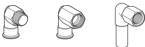
Afbeelding 10: Geberit Mapress Therm en Geberit Mapress rvs overgangsknie 90°
