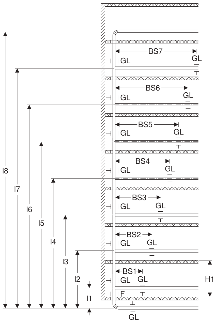
Afbeelding 39: Stijgleiding met fixpunt onder: geleiding van de uitzetting naar boven
