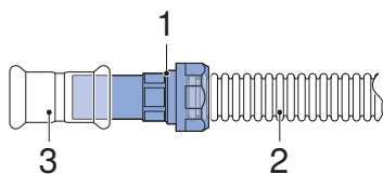
Afbeelding 28: Overgang naar ribbelbuizen
