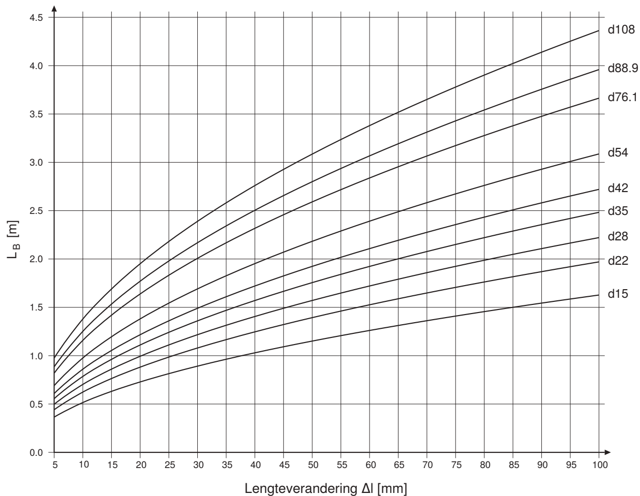
Afbeelding 45: Buigbeenlengte L_B voor Geberit Mapress Therm
