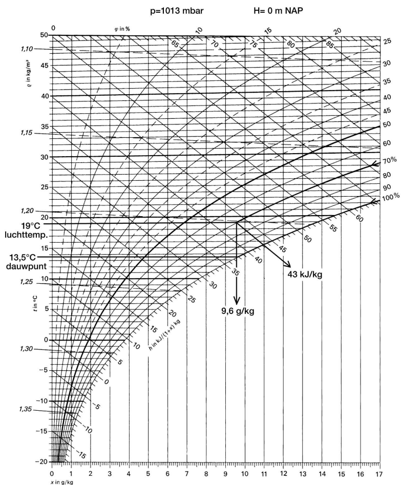
Afbeelding 5: x (Mollier)-diagram
