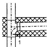
Afbeelding 37: Uitvoering met gelijkzijdig T-stuk (verlopende T-stukken moeten verankerd worden)
