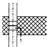
Afbeelding 36: Uitvoering met kraagbus
