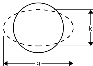
Afbeelding 46: Ovaliteit van lasdelen
